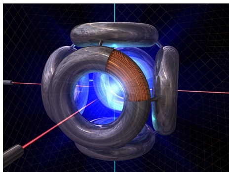
Polywell WB-1 mit würfelförmiger Spulenordnung
