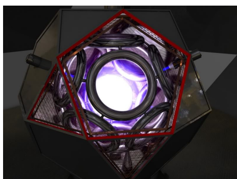
Polywell WB-6 mit Dodekaeder Spulenordnung
